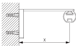
Smart Fix con asola SG 11206 - SG 11208: Necessaria vite SG 10492 (M4x8).
