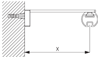
Smart Fix squadrato con asola SG 11216 - SG 11218: Necessaria vite SG 10492 (M4x8).
