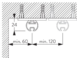
Supporto SG 6124
