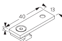
SG 6151 Set supporto a soffitto 3 mm
