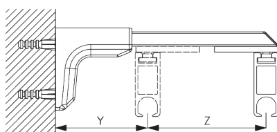
Doppio sistema: Smart Fix universale SG 11155 - SG 11156 e SG 6151: Necessaria vite SG 11127 (M4x10) e dado SG 11148.
