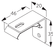
SG 2343 Supporto universale 46 mm
