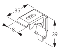
SG 2302 Supporto universale
