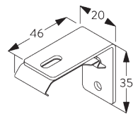
SG 2343 Supporto universale 46 mm
