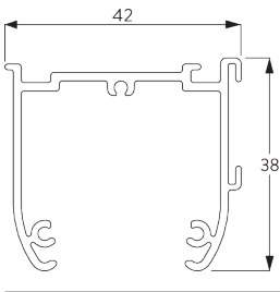
SG 2321 Profilo
