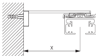
Smart Fix squadrato SG 11212 - SG 11214 e supporto girevole SG 3044: Necessaria vite SG 10395 (M4x6).
