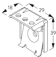
SG 8201 Supporto
